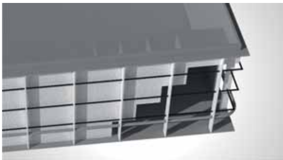
klatka schodowa zaprojektowana do podbetonowania
